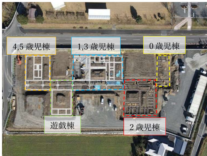
0歳児棟・2歳児棟…基礎の鉄筋組立て作業
