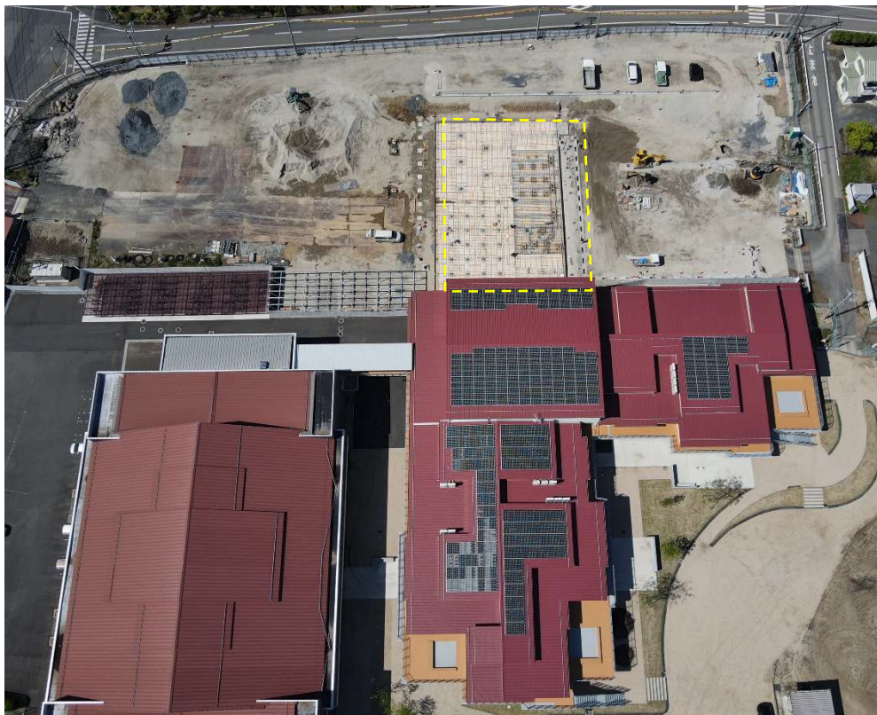
中学校の北棟の工事の様子（5月14日撮影）
