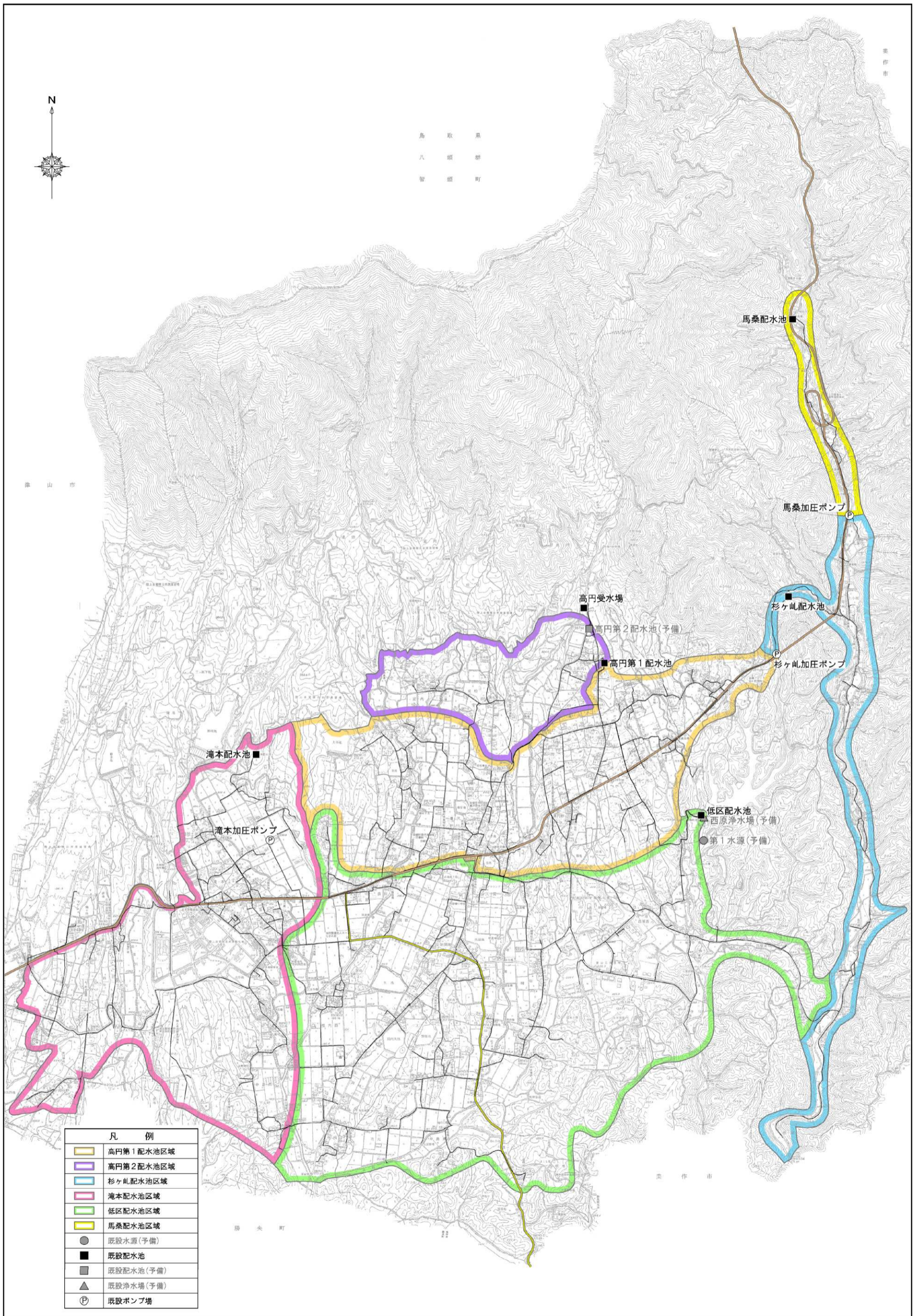
図 2-5 水道施設一般平面図
